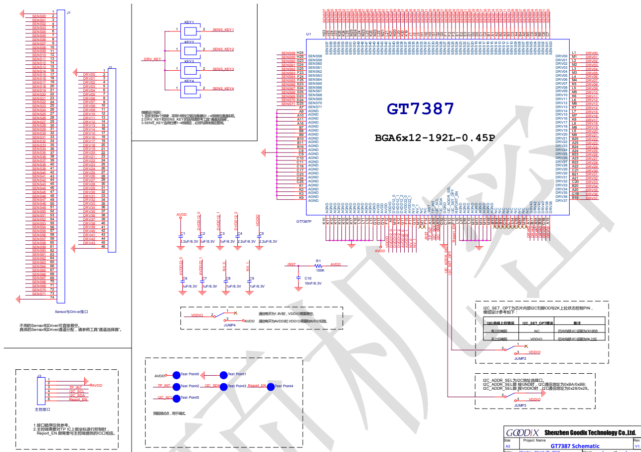
GT7387 参考应用电路图
